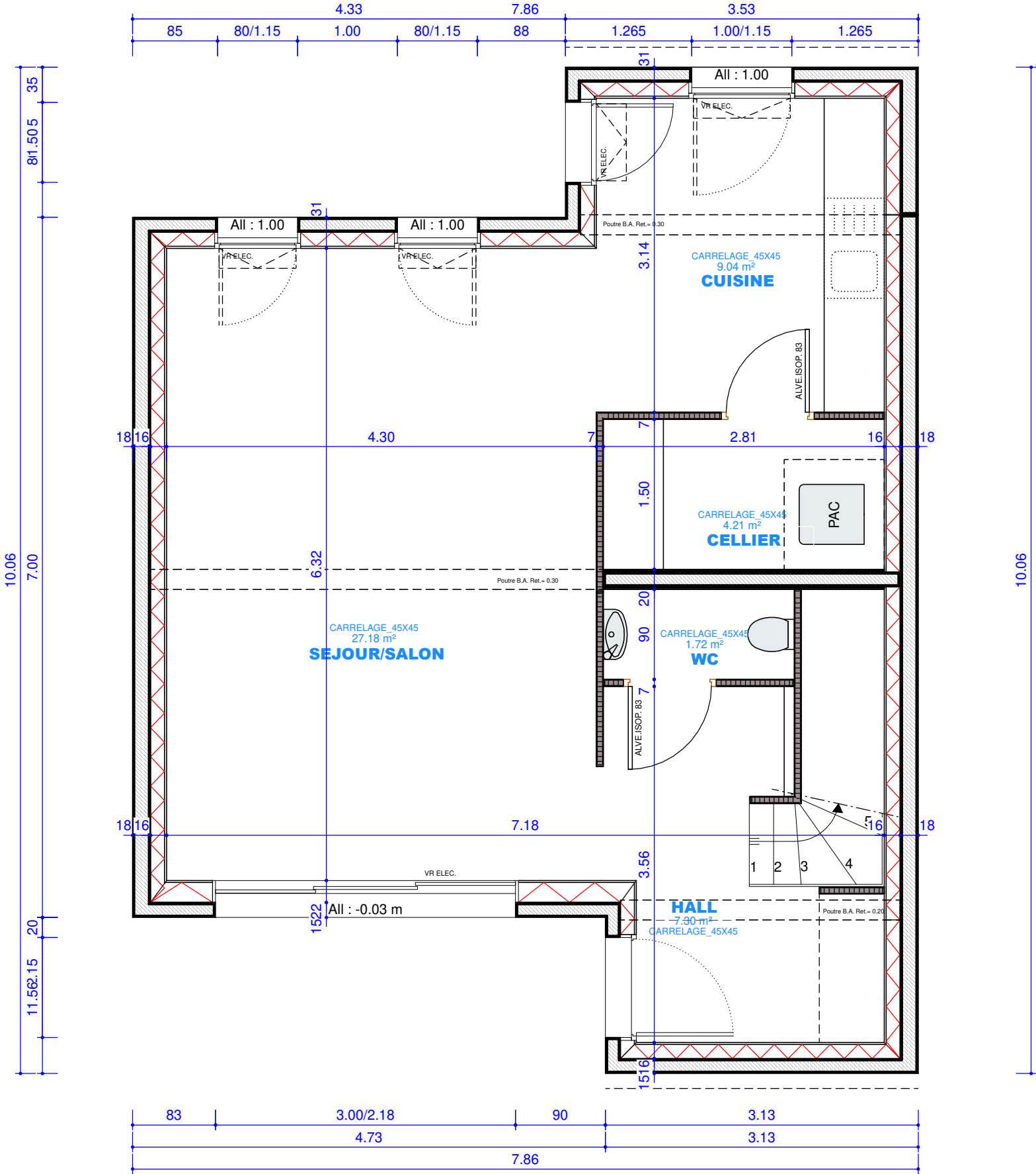
VUE EN PLAN DU REZ DE CHAUSSEE
